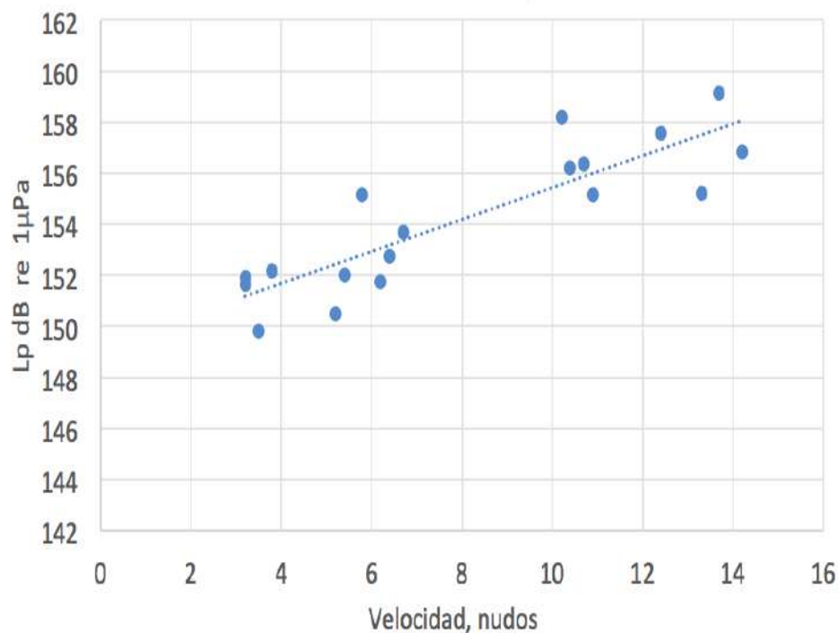
Emisión de ruido subacuático Embarcación 60 Hp
