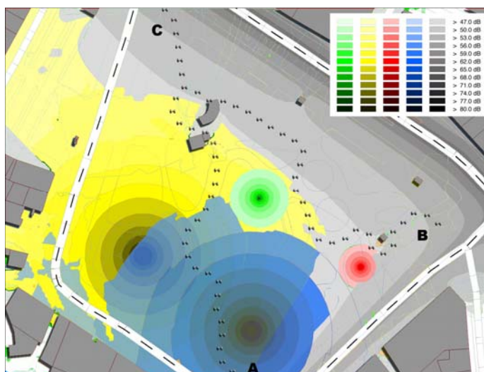
Mapa sonoro global
