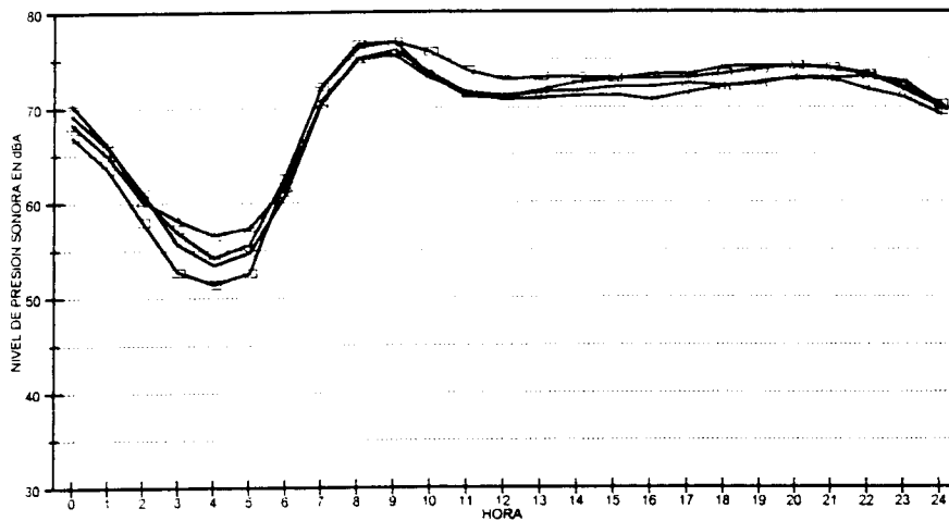
CICLO HORARIO DE RUIDO EN DIAS HABILES PUNTO BASE AMERICO VESPUTIO
